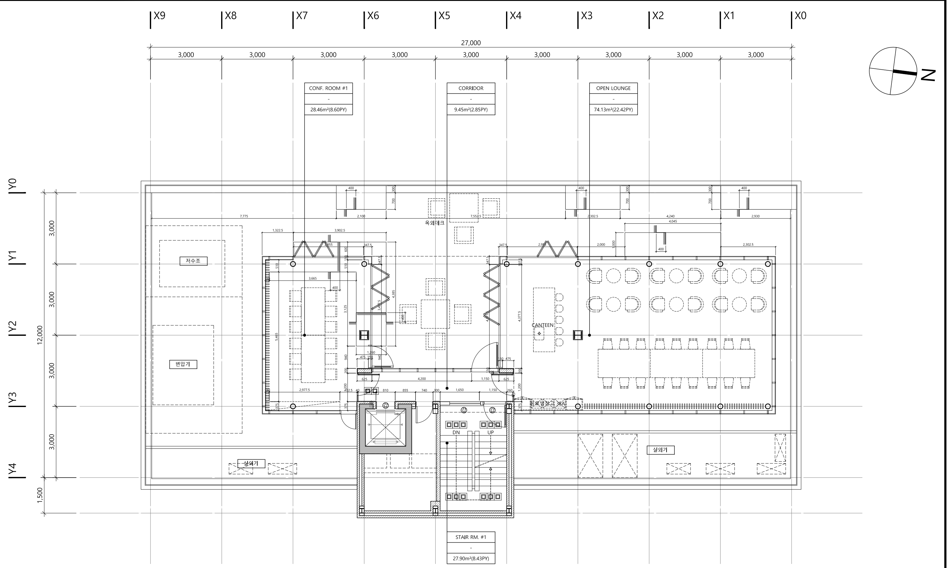
1 A-121 5F FLOOR PLAN SCALE : 1 / 100
